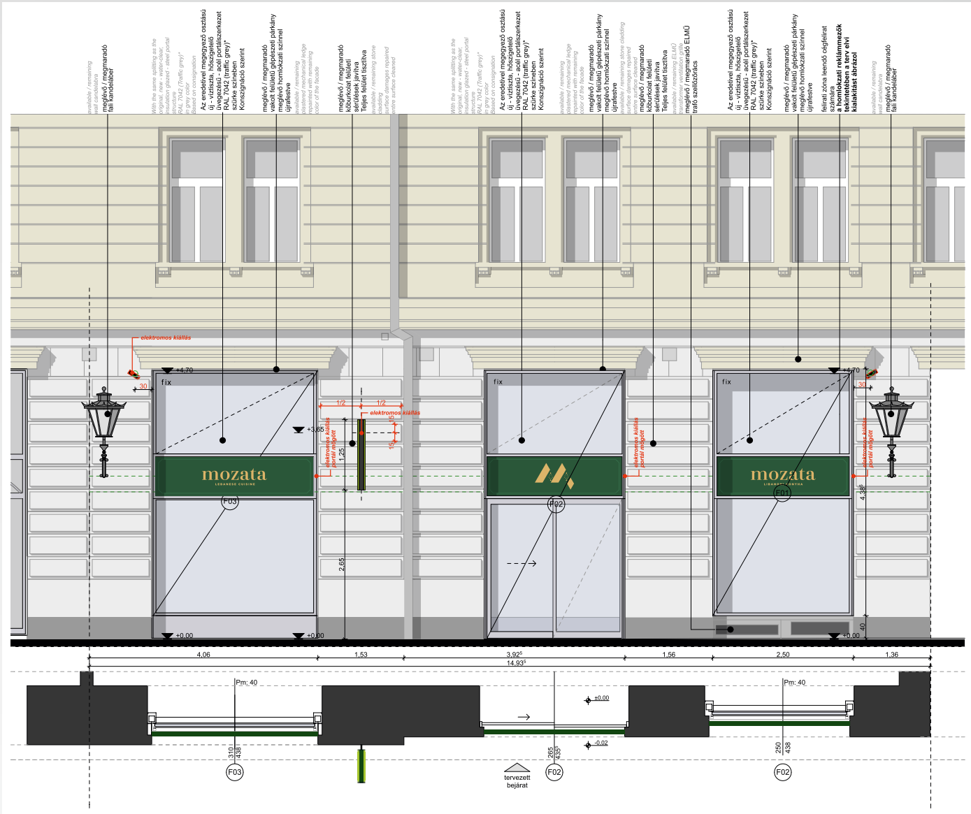
ÉPÍTÉSI ENGEDÉLYEZETT HOMLOKZATI RAJZ
